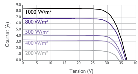
Caractéristiques courant/tension en fonction de l'éclairage et de la température du module.
